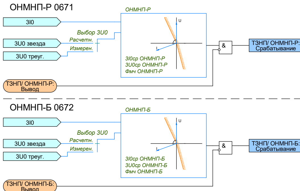
Рисунок 2.24 – Функциональная схема логики ОНМП
